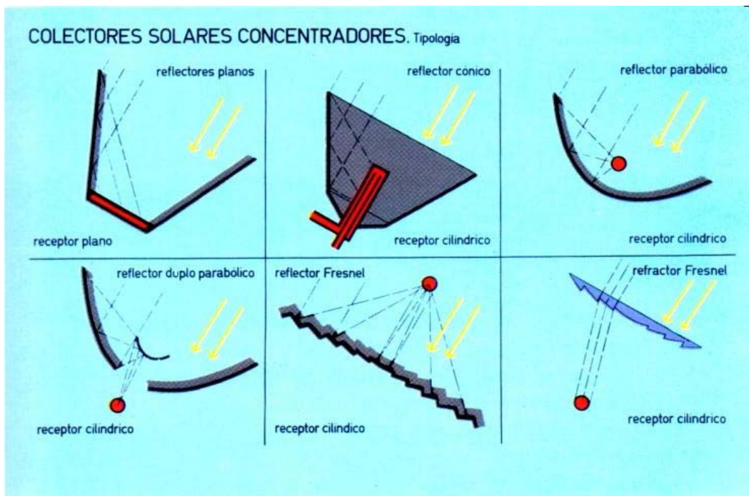
Concentradores catóptricos e dióptricos
