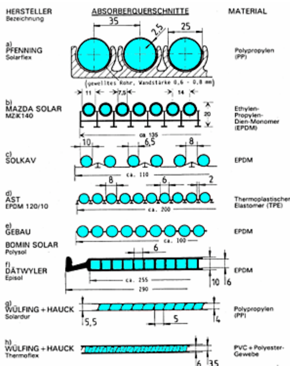
Exemplos de absorvores (extra3do do CD ROM MULTISOL)
