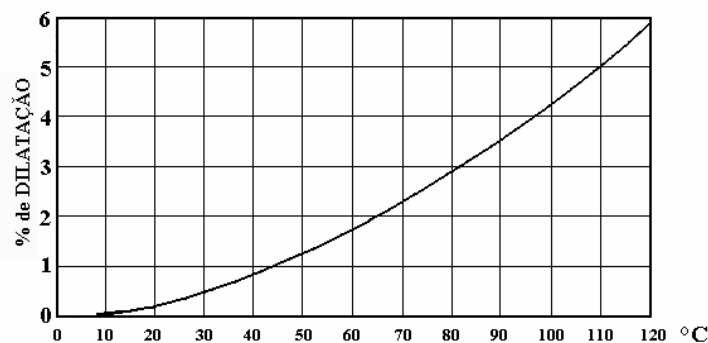
Dilatação da água em função da temperatura (Referência volume a 4°C)
