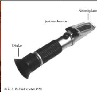
Bild 1 Refraktometer R20
