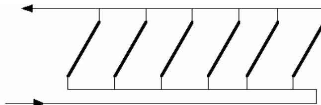
Ligação em paralelo com alimentação invertida.
