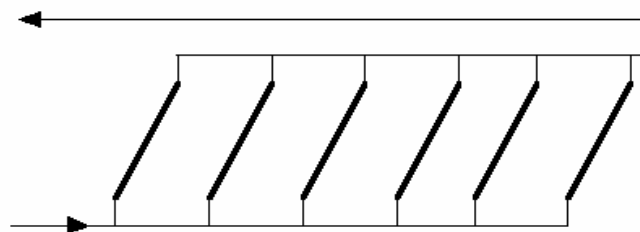
Ligação em paralelo com retorno invertido.
