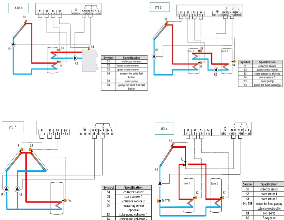
(Modos de funcionamento do controlador DeltaSOL BS Plus)
