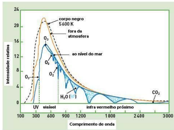
Espectro da radiação solar, que chega à superfície da Terra (nível do mar). Comparação com a radiação fora da atmosfera. (As indicações de O 3 , O 2 , H 2 O e CO 2 , indicam a absorção do espectro por esses compostos)
