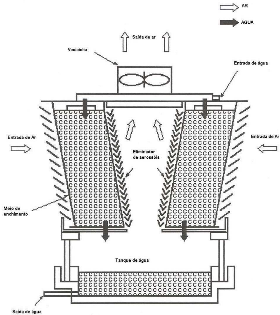
Figura 7: Torre de arrefecimento ou refrigeração para edifícios de grande dimensão (Department of Human Services “Guidelines for Control of Legionnaires Disease”, Victoria State Austrália)
