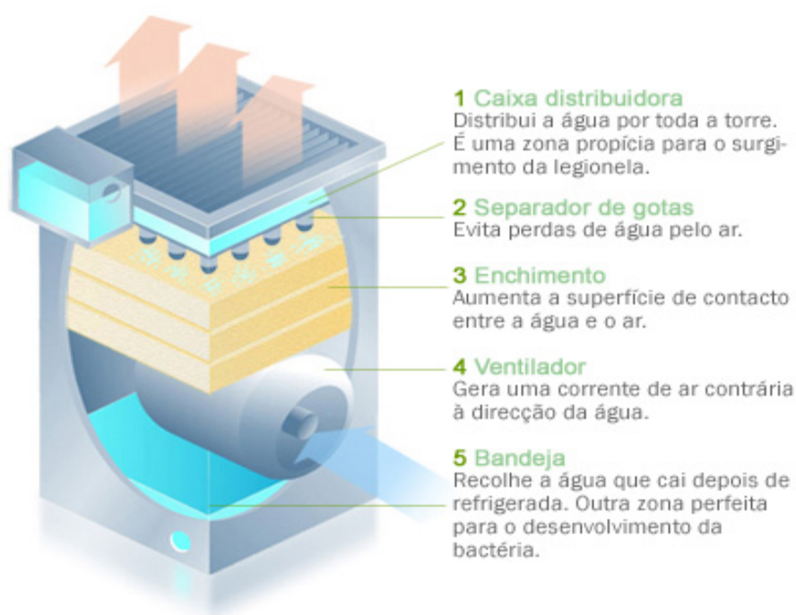
Figura 6: Descrição das partes de uma instalação
